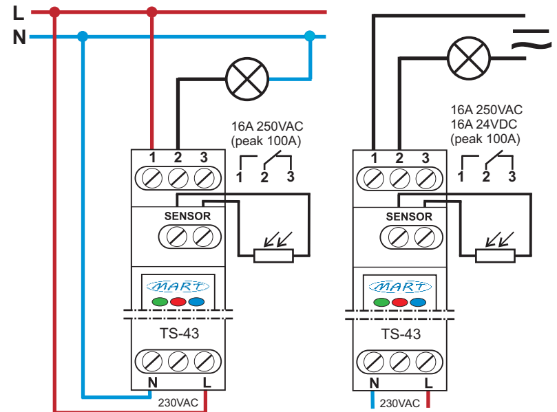
Rys. 2. Schematy podłączenia AUTOMATU ZMIERZCHOWEGO TS-43-2.
