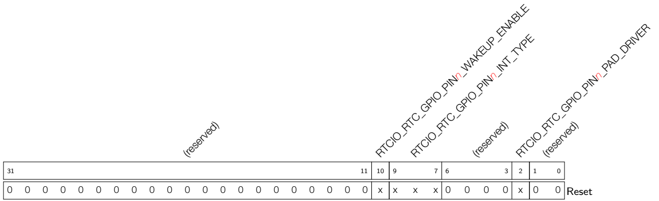
Register 4.45: RTCIO_RTC_GPIO_PIN n _REG ( n : 0-17) (28+4* n )
