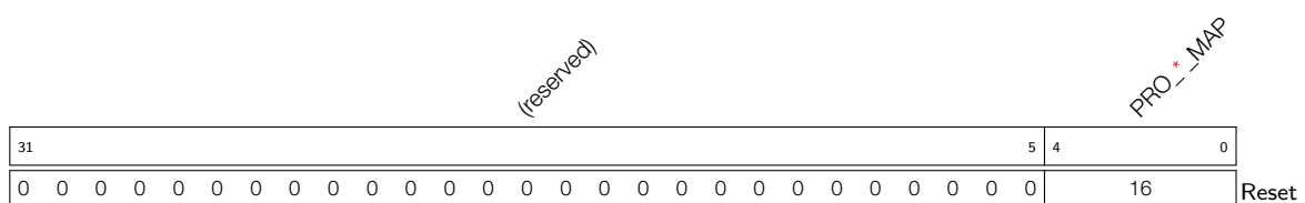
PRO*_MAP Interrupt map. (R/W)
