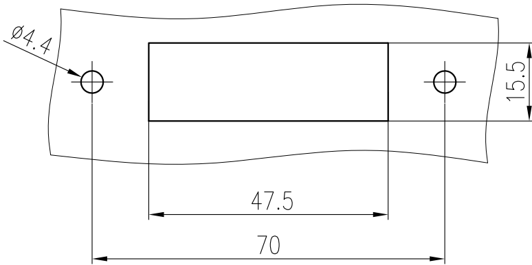
面板开孔图
