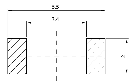
P. C. B. Land Patten
