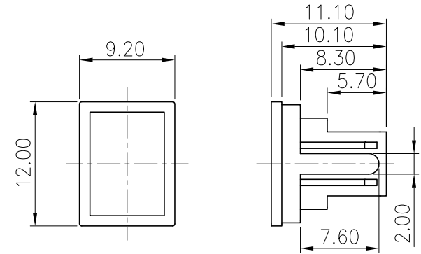
防尘帽图示
