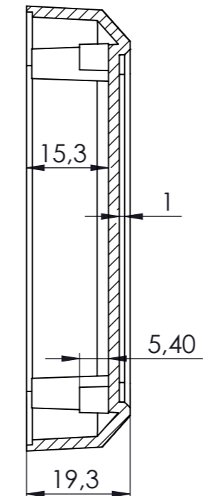
KESIT A-A
