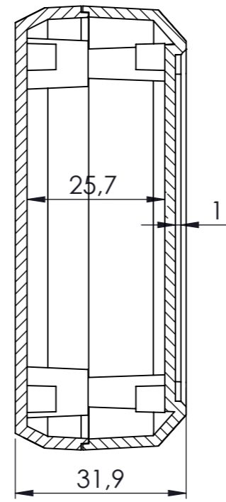
KESIT A-A
