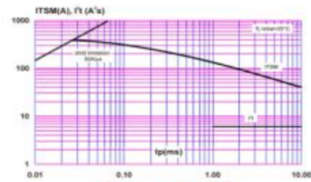
6、 I_{TSM}-I^2t-t 曲线
