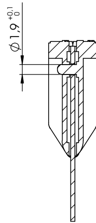
SEZIONE A-A
