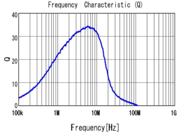
■ LQM21PN1R0MC0 Q
