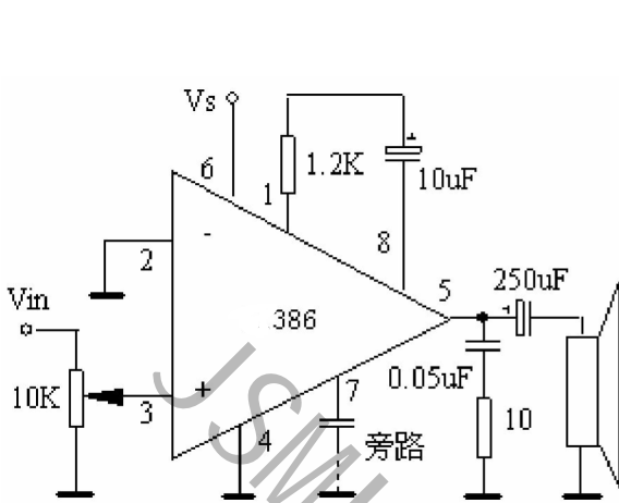
图3 放大器增益=50
