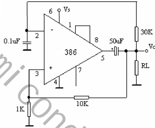
图6 方波振荡器
