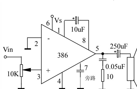
图2 放大器增益=200
