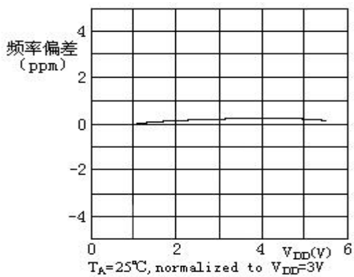
频率偏差与 V_{DD} 的关系图
