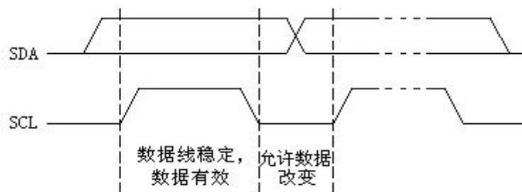
图12. I2C总线上的位传送
