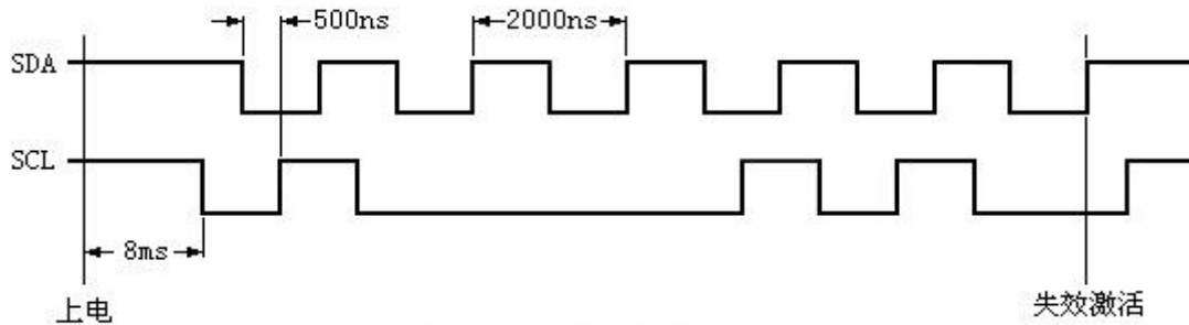
图9. POR失效时序图
