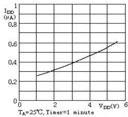
CLKOUT=32.768kHz, I_{DD} 与 V_{DD} 的关系图
