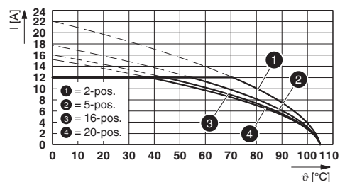
Typ: FKCS 2,5/...-ST-5,08 z MSTBVA 2,5/...-G-5,08
