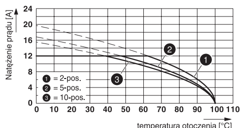
Typ: TVMSTB 2,5/...-ST-5,08 z MSTBVA 2,5/...-G-5,08
