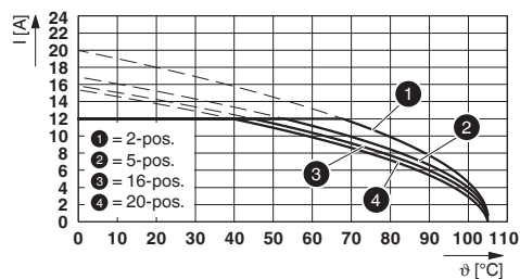
Typ: FKCT 2,5/...-ST-5,08 z MSTBVA 2,5/...-G-5,08
