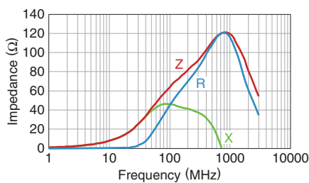
MPZ1608Y600BTD25
