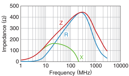
MPZ1608R391ATD25
