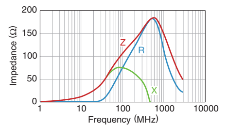
MPZ1608Y101BTD25
