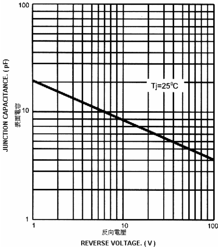
FIG. 3- 表面電容(典型值) FIG. 3 - TYPICAL JUNCTION CAPACITANCE
