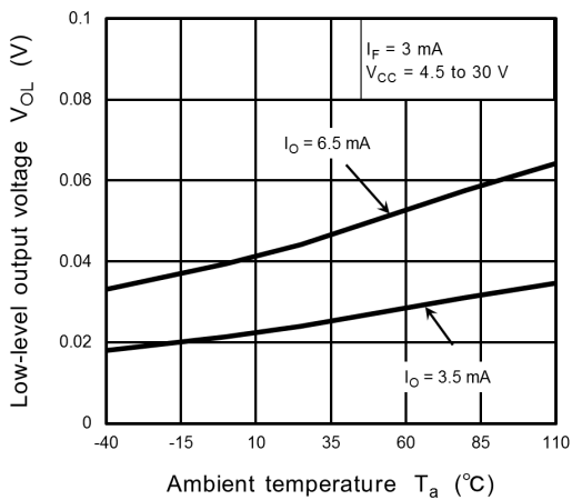
Fig. 12.2.5 V_{OL} - T_a
