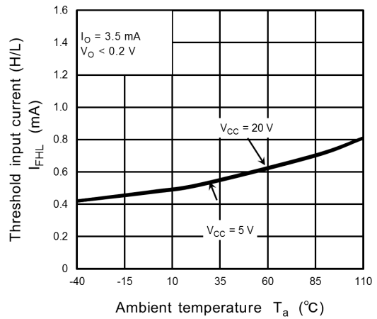
Fig. 12.2.2 I_{FHL} - T_a
