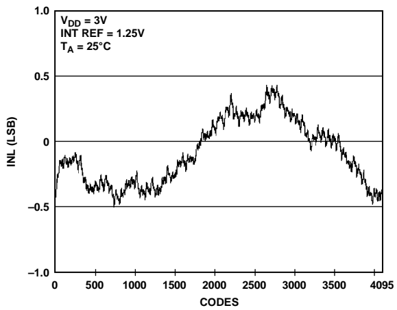
Figure 20. INL AD5628-1
