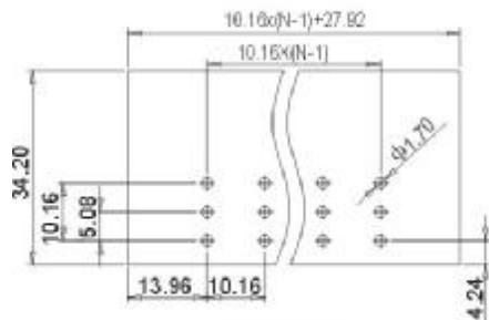
PCB LAYOUT(REF)
