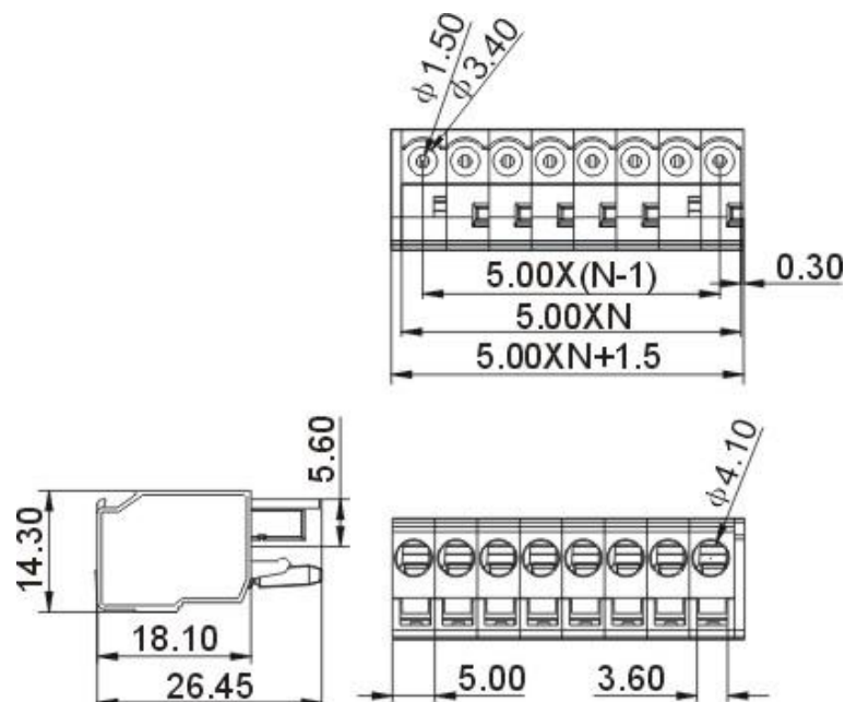
8EDGK-5.0 8EDGK-5.08
