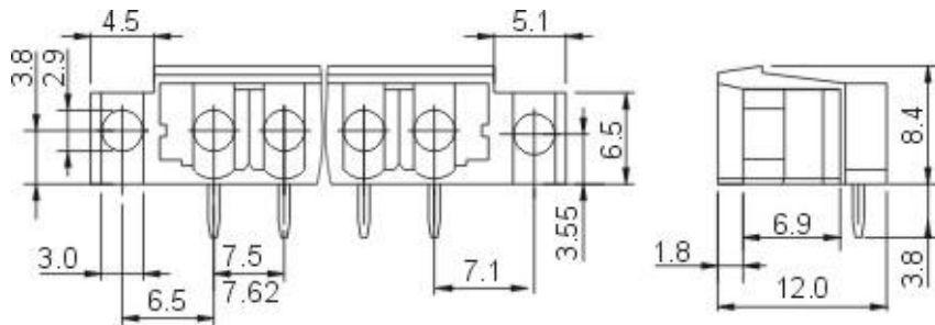
8EDGRMA-7.5 8EDGRMA-7.62
