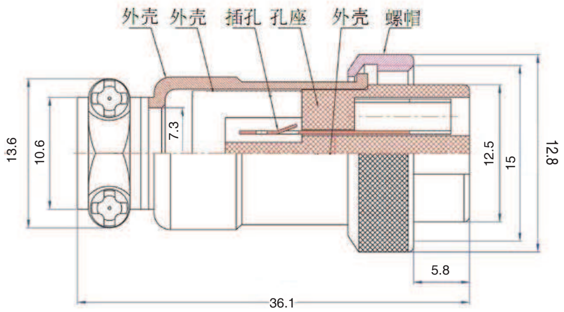
GX16头尺寸图
