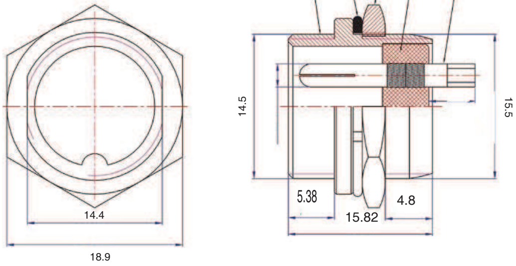
GX16座尺寸图
