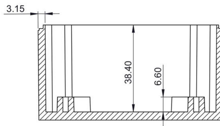
PRZEKRÓJ A-A
