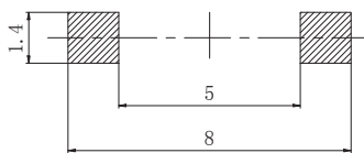
安装尺寸图
